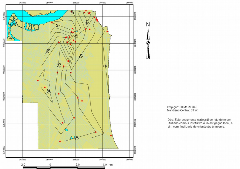
Figura 1. Carta da Superfície Superior do Aquitardo Potengi-Barreiras.
