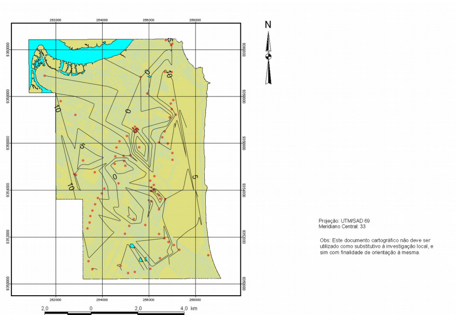
Figura 1. Carta da Superfície Superior do Aquitardo Potengi-Barreiras.
